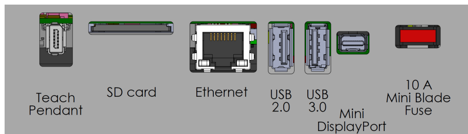
Externa anslutningsportar.
