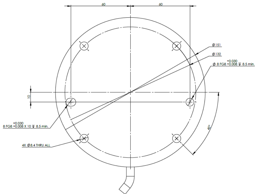
1.1: Undersidan av robotbasen
